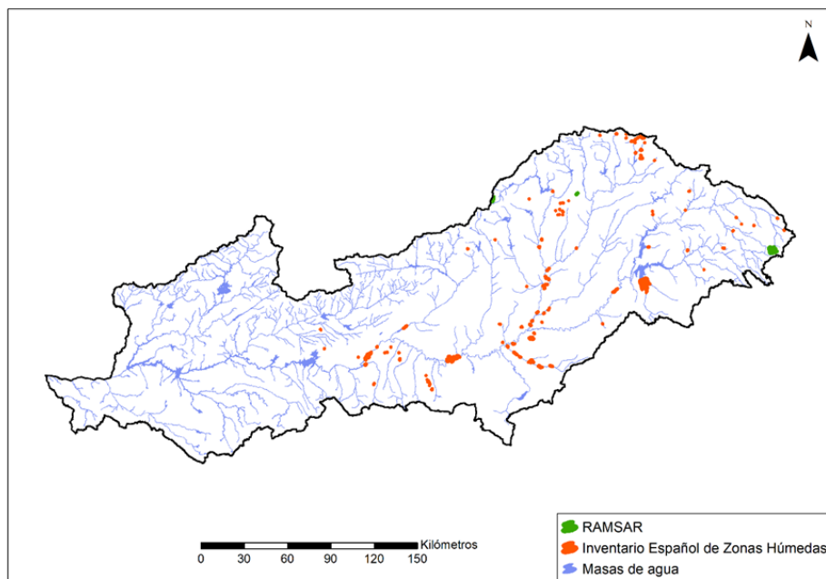
Figura 8. Zonas húmedas en la cuenca del Tajo
